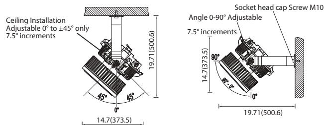
Yoke
